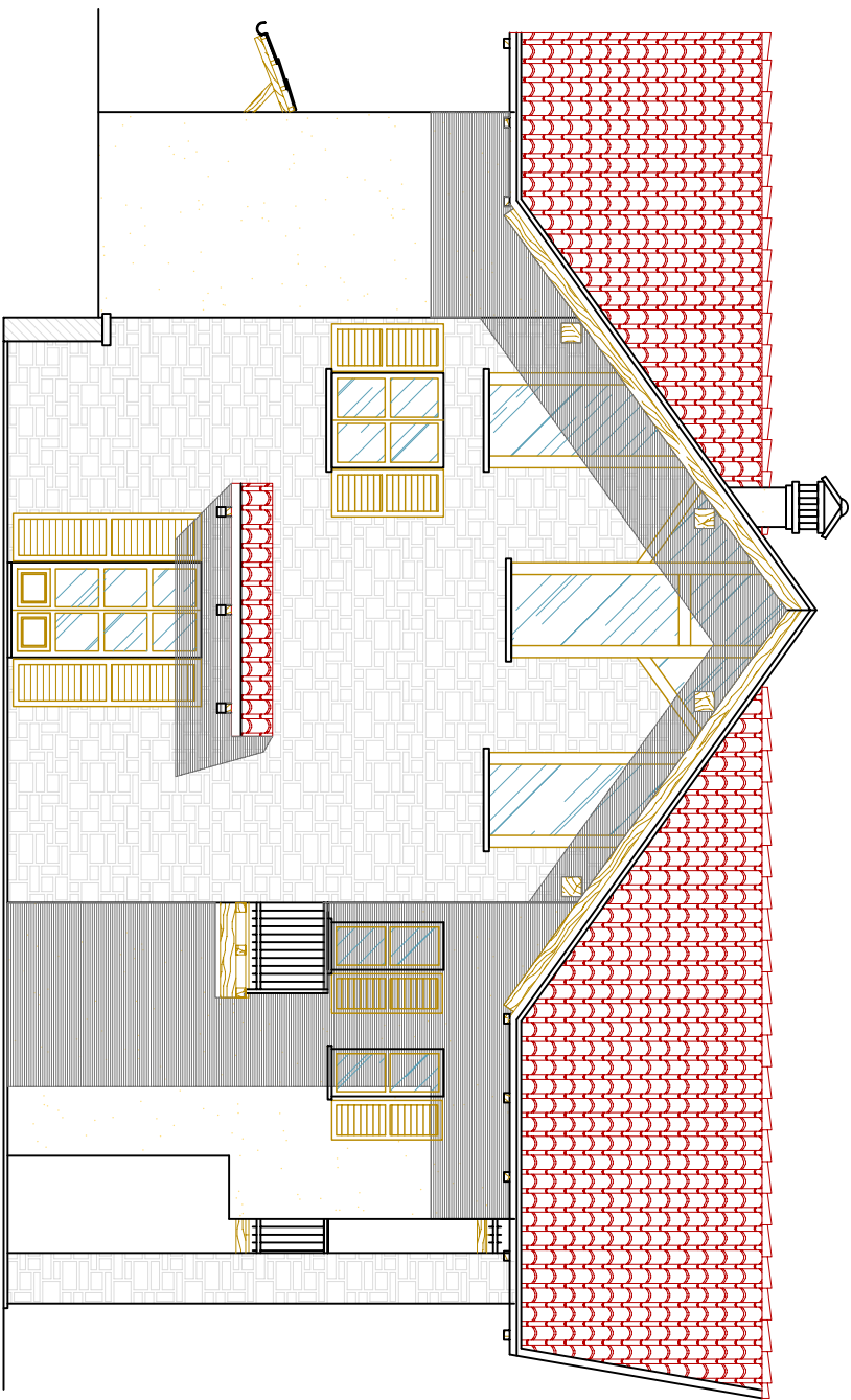
Prospetto Ovest
